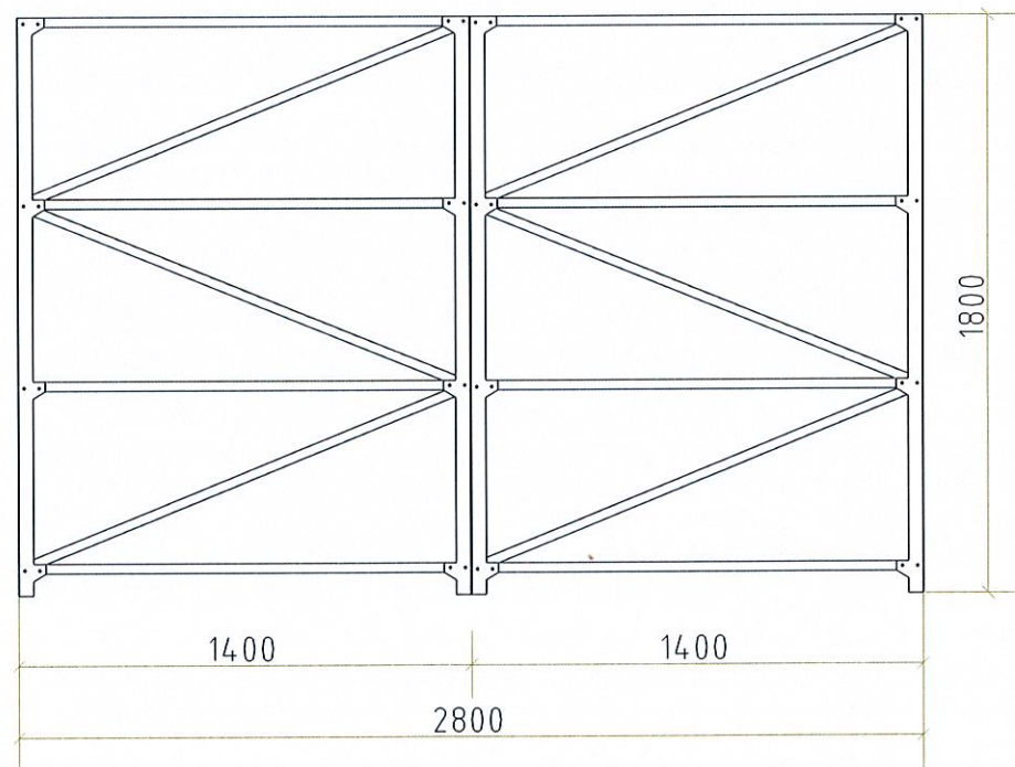
2号冷库货架3正立面图 1:30
