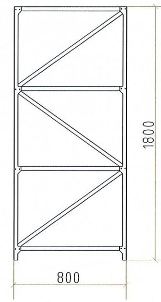
4号冷库货架侧立面图 1:30
