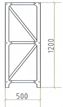
1号冷库货架3侧立面图 1:30
