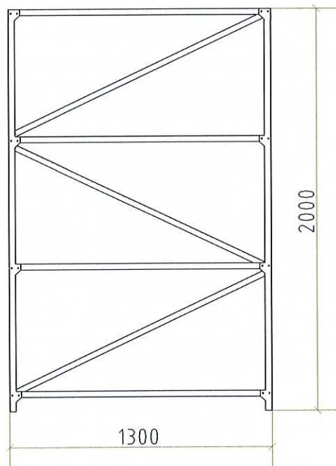
5号冷库货架2正立面图 1:30
