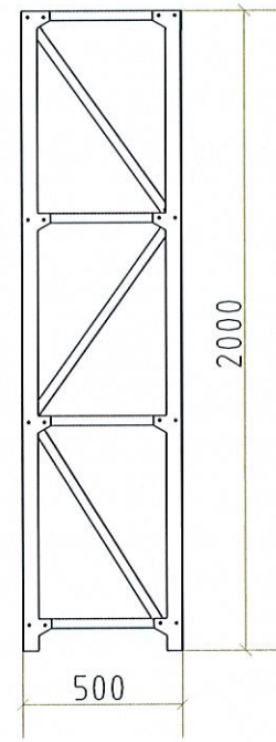
5号冷库货架2侧立面图 1:30
