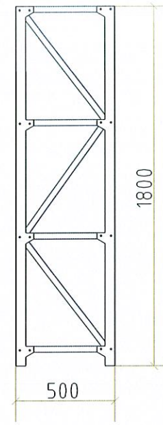
2号冷库货架2侧立面图 1:30
