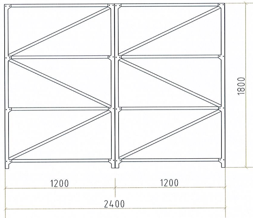
1号冷库货架2正立面图 1:30
