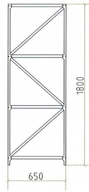
4号冷库货架1正立面图 1:30
