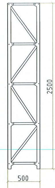
6号冷库货架1侧立面图 1:30
