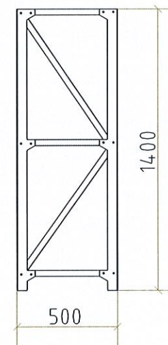
4号冷库货架3侧立面图 1:30
