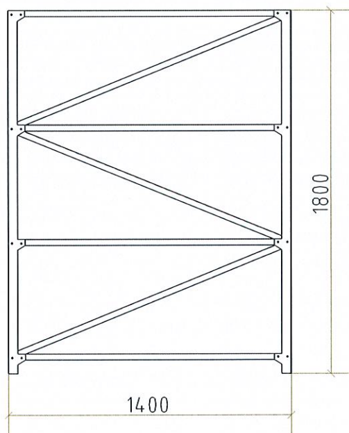
3号冷库货架1正立面图 1:30
