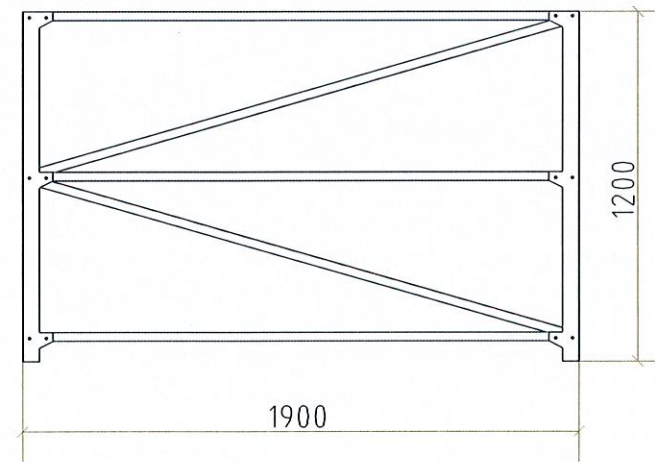
1号冷库货架3正立面图 1:30
