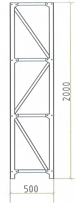
4号冷库货架2侧立面图 1:30
