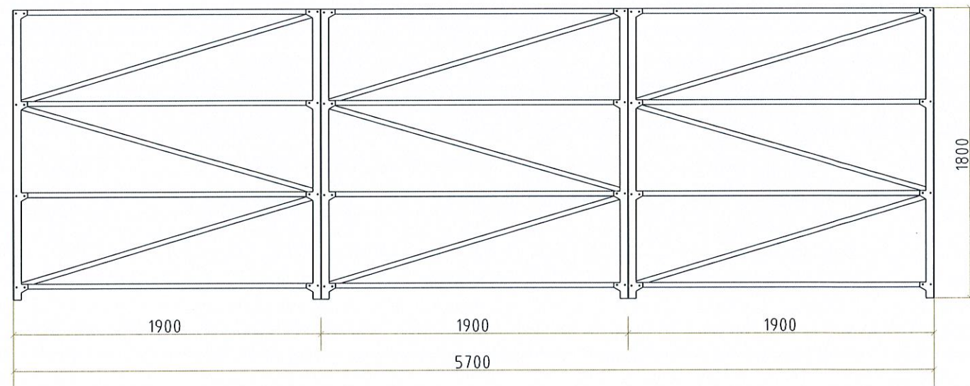
6号冷库货架3正立面图 1:30
