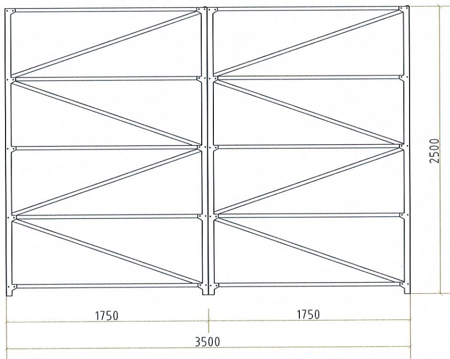
6号冷库货架2正立面图 1:30
