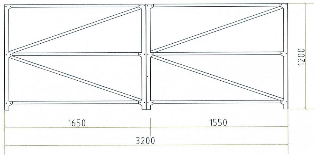
2号冷库货架1正立面图 1:30
