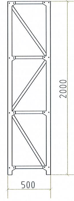
5号冷库货架3侧立面图 1:30
