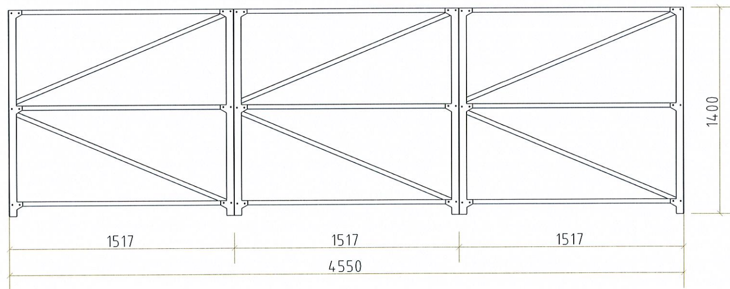
4号冷库货架3正立面图 1:30
