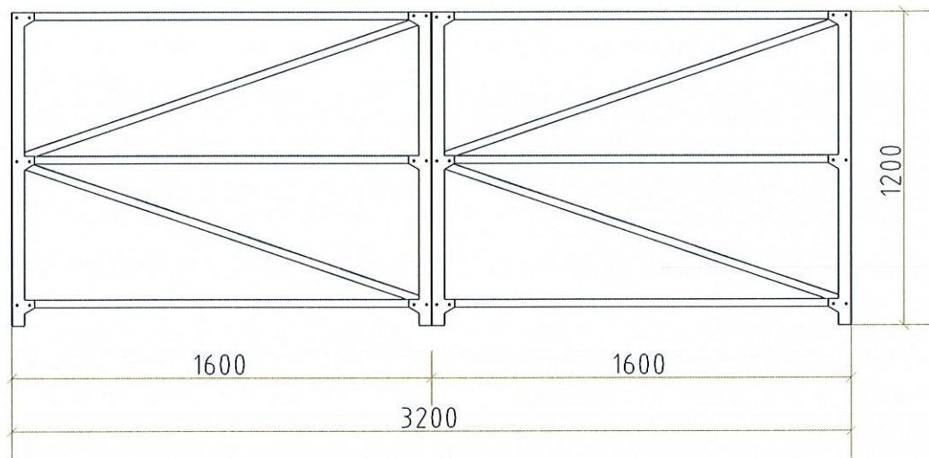
1号冷库货架1正立面图 1:30
