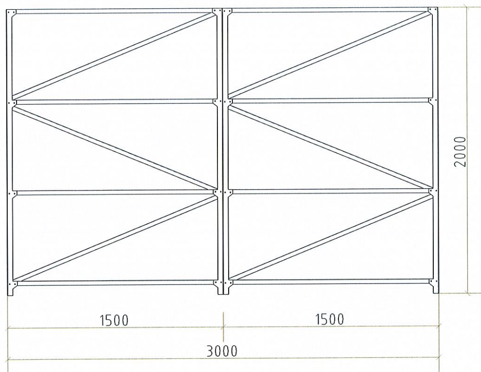
4号冷库货架1正立面图 1:30
