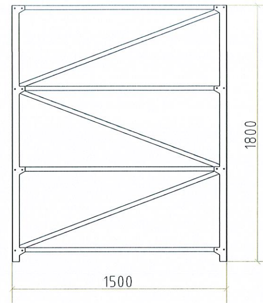
2号冷库货架2正立面图 1:30
