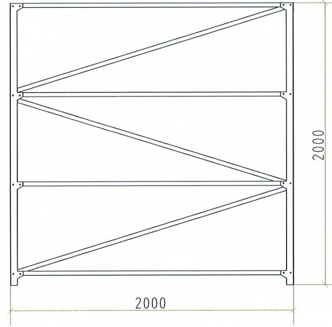
5号冷库货架3正立面图 1:30
