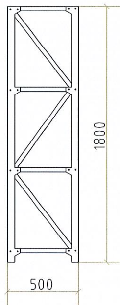
3号冷库货架侧立面图 1:30
