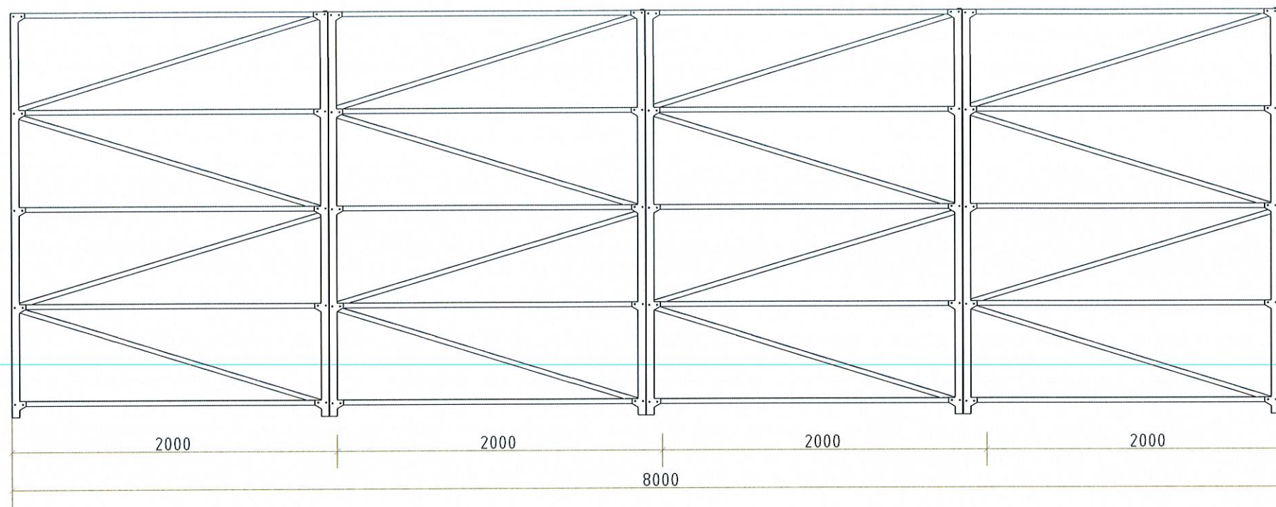
6号冷库货架1正立面图 1:30
