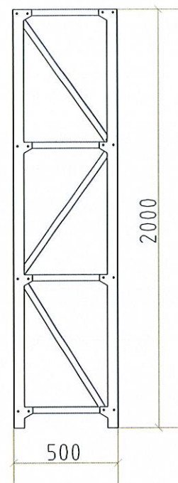
4号冷库货架1侧立面图 1:30
