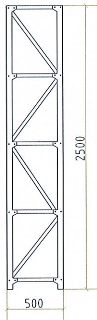
6号冷库货架2侧立面图 1:30
