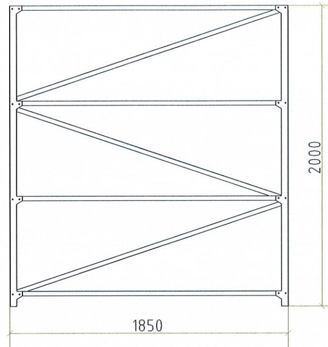
4号冷库货架2正立面图 1:30
