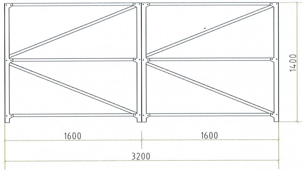
5号冷库货架1正立面图 1:30
