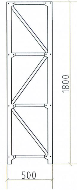
1号冷库货架1侧立面图 1:30
